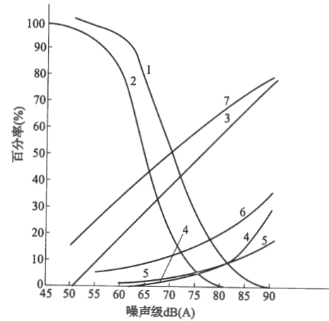
图1 洁净厂房噪声分布与评价图
